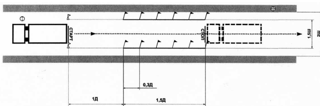
Рис. 10. Упражнение №10 «Прямолинейное движение ходом»
