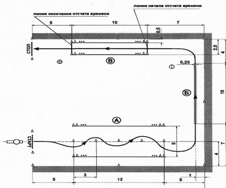
Рис.2. Упражнение №2 «Змейка», «колейная доска», движение с малой скоростью» Контрольная таблица №2
