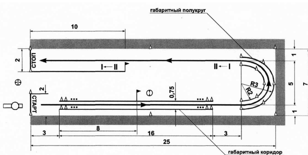
Рис.1. Упражнение №1 «Габаритный коридор, «габаритный полукруг», разгон-торможение»
