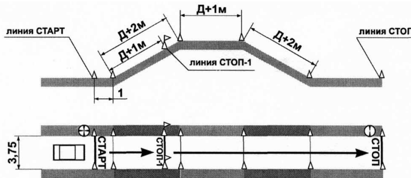
Рис.4. Упражнение №4 «Остановка и трогание на подъеме»
