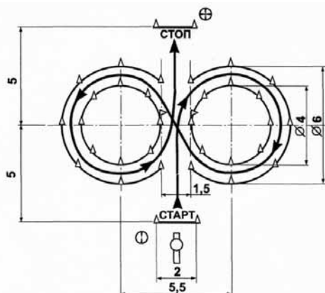
Рис.3. Упражнение №3 «габаритная восьмерка»
